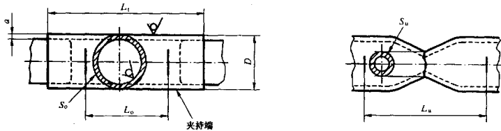
图 14 管段试样(见附录 D)
