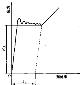
图6 屈服点延伸率( A_e )
