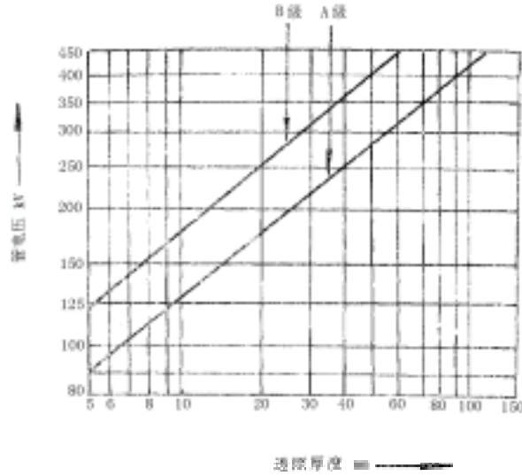
图 1 管电压与透照厚度关系
