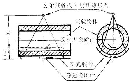
图 4 管状铸件透照配置（双壁单层透照法）
