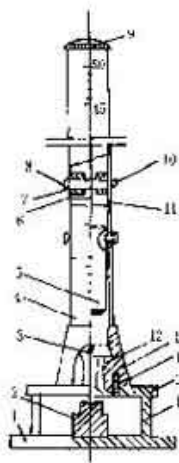
冲击试验器
