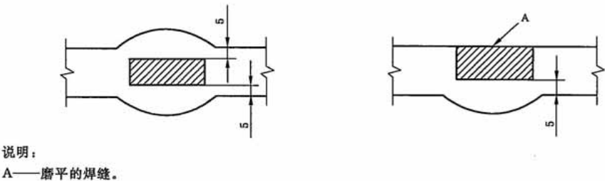
图 1 焊缝中显示的位置
