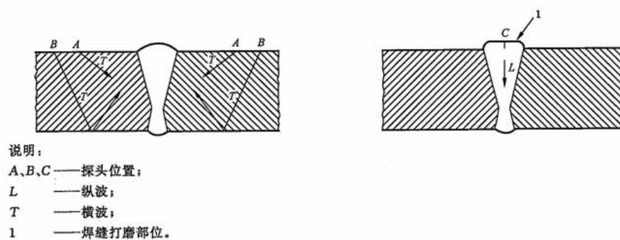
图 B.1 检测方向示例
