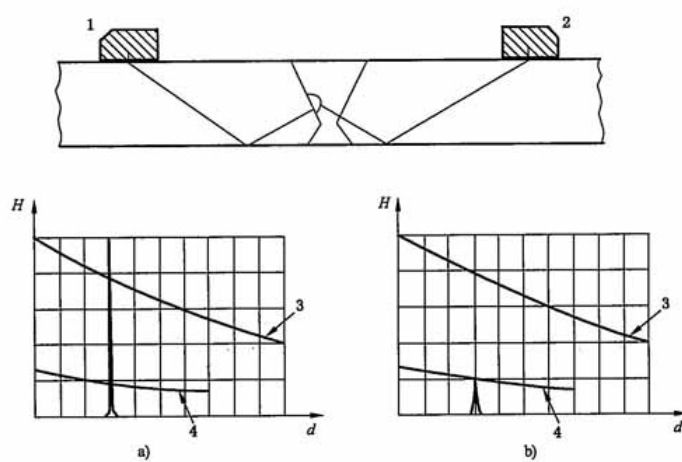
图 B.1 检测方向示例
