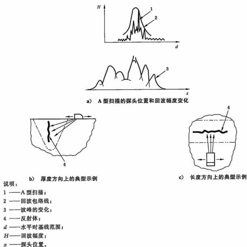
图 C.4 超声响应的波形 4
