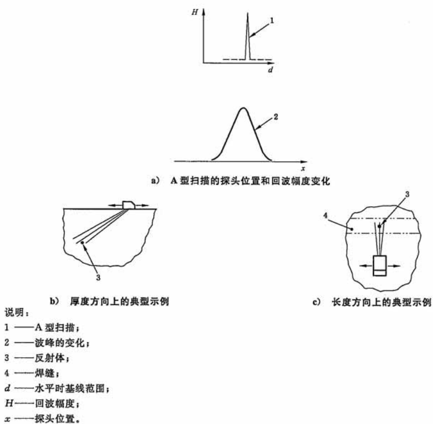
图 C.1 超声响应的波形 1
