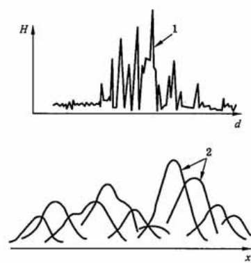
a) A 型扫描的探头位置和回波幅度变化
