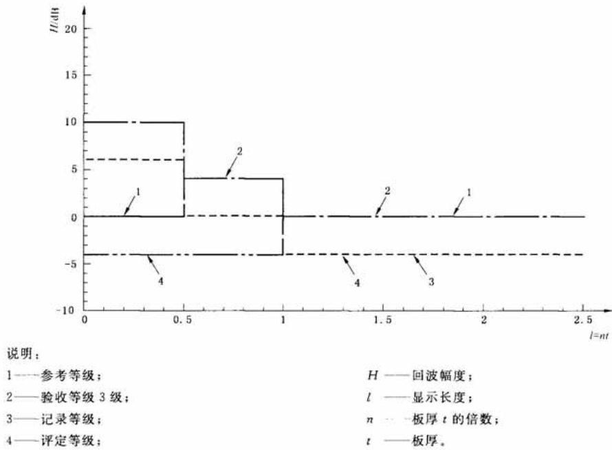
图 A.9 适用于板厚 15 mm~100 mm 的平底孔技术(技术 2)的等级 验收等级 3 级
