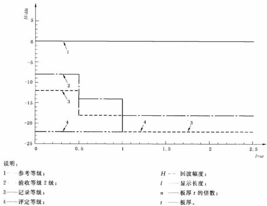
图 A.8 适用于板厚 15 mm~100 mm 的串联式技术(技术 4)的等级 验收等级 2 级
