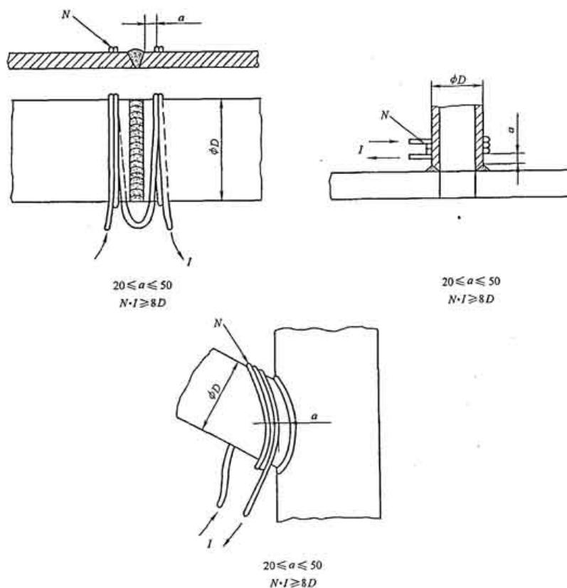
图 6 柔性电缆或线圈的典型磁化技术（适用于检测纵向裂纹）
