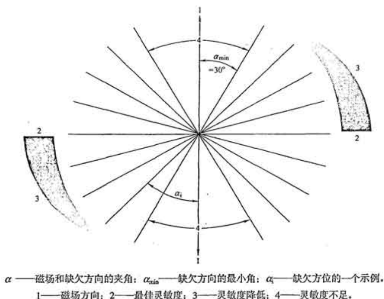
图 1 可检测出的缺欠方向
