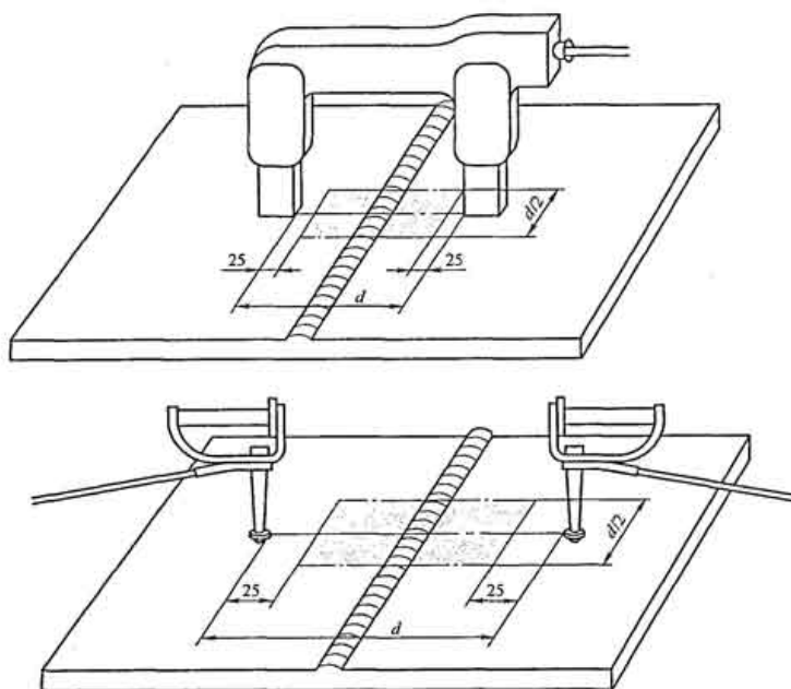
图2 磁轭和触头磁化的有效检测区域（阴影）示例
