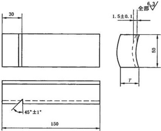
图 1 GD-I 对比试块
