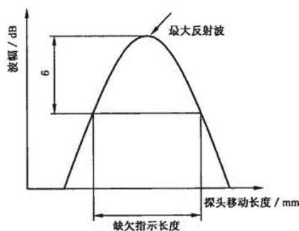
图 6 6 dB 测长法
