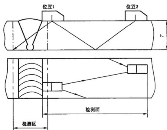
图 2 检测和探头移动区
