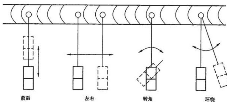
图 4 四种基本扫查方法
