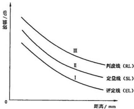
图5 距离-波幅曲线示意图
