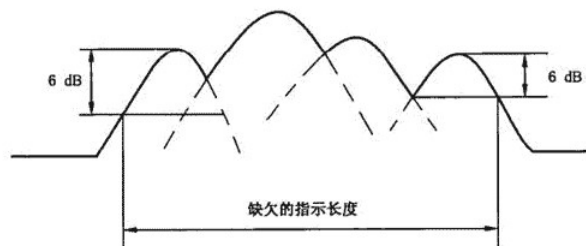
图 7 端点 6 dB 测长法
