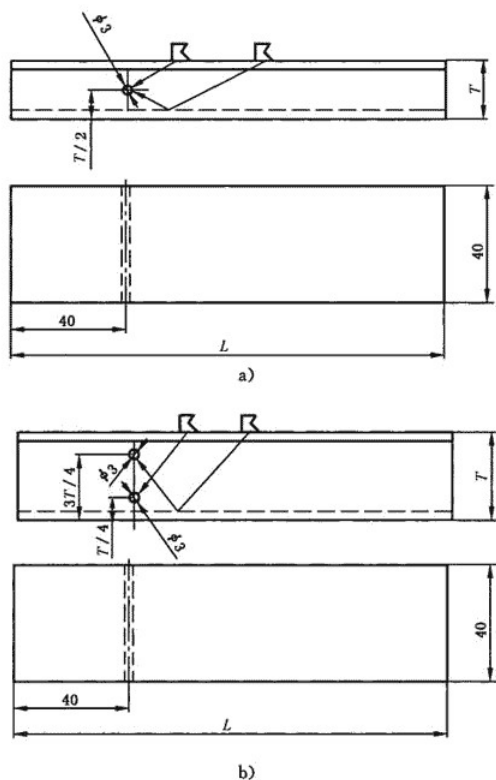
图 A.1 补偿量测量试块
