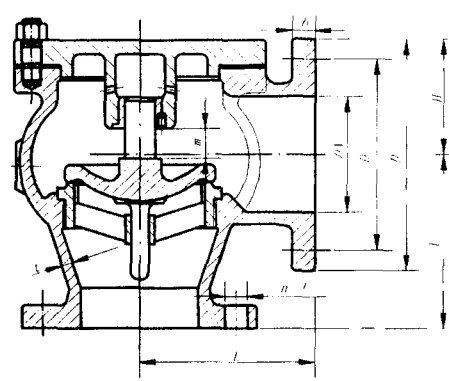
图2 BJ型止回阀
